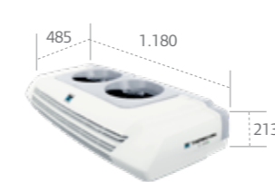
Condensatore C-450e
